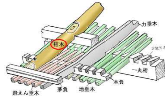
1-①-ロ 不足の榑木(ハネギ)の補充。
